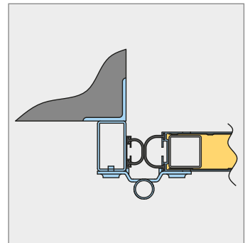
Dichtungssystem
